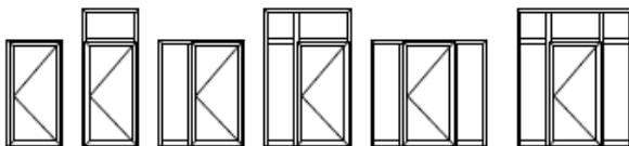
Į IŠORĘ ATIDAROMOS DURYS
